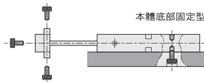
滑塊可由三方向固定
