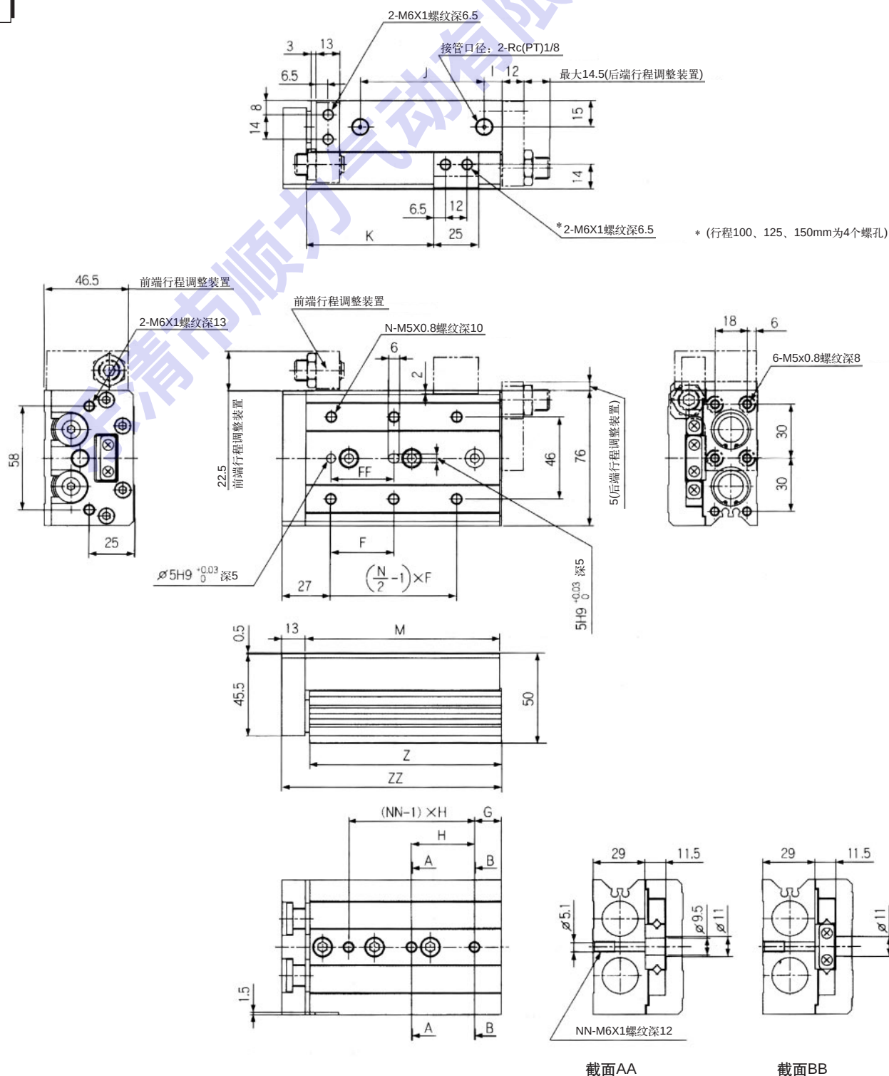
截面AA
